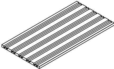
Core DRY Zuführplatte / 5 Streifen (1000 x 500 mm)
